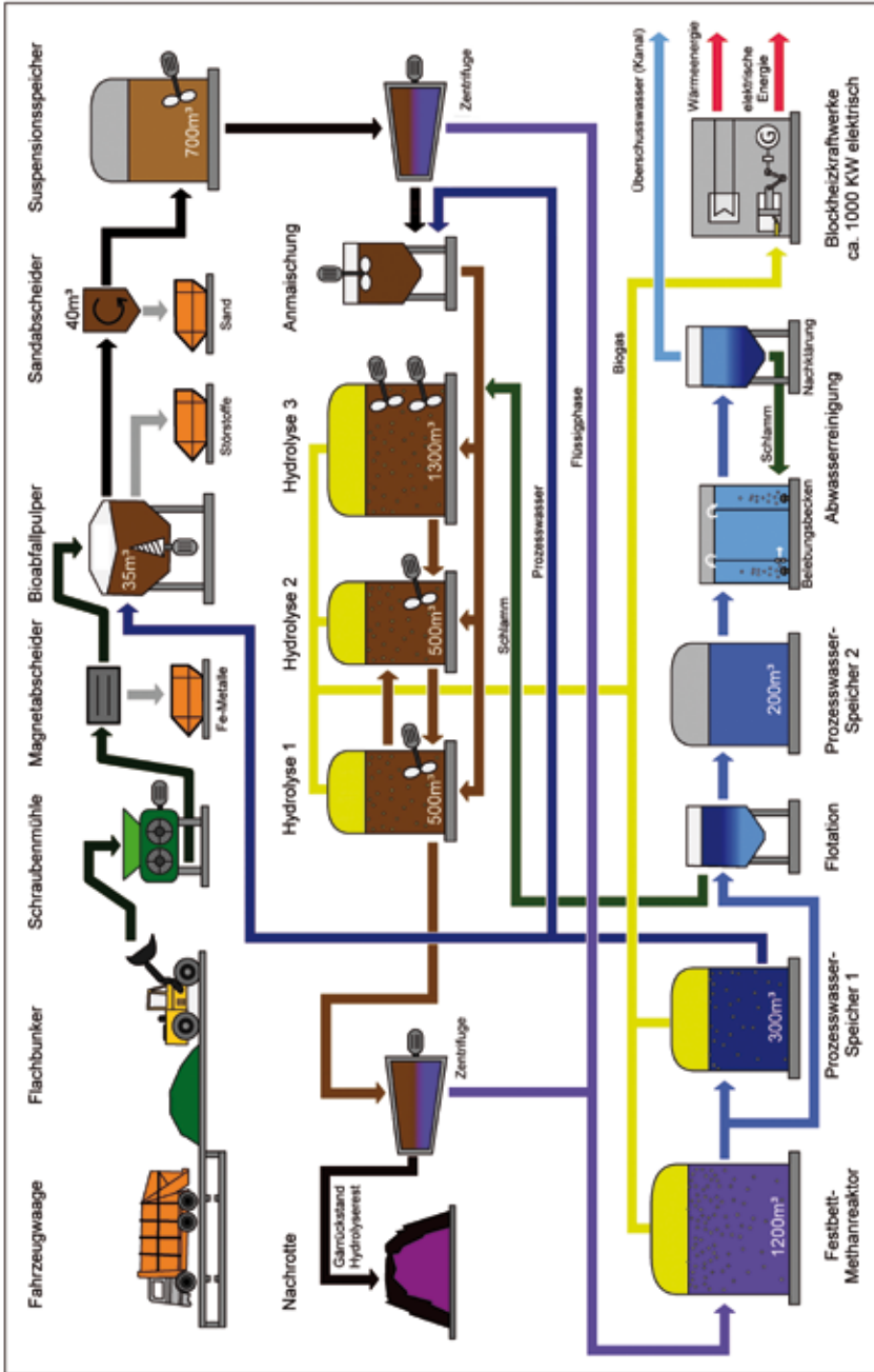
So funktioniert die Biovergärungsanlage in Brunenthal-Kirchstockach. Quelle: Ganser Entsorgung GmbH & Co. KG
